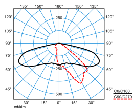
Cuvia40-AB2L2LR-S3-22-722-ET-CAE-26 (CLO end value)
