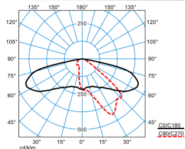
Cuvia40-AB2L2LR-S3-22-722-ET-CAE-26 (CLO initial value)
