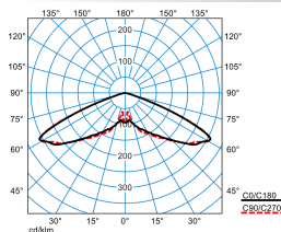
Publisca P1W-RB6L-LRA/4600-730 6G1S ET (CLO initial value)
