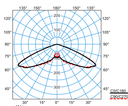
Publisca P1W-RB6L-LRA/4600-730 6G1S ET (CLO end value)
