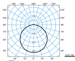
Olisq RWD4 DW 40-830 ET + Olisq RWD4 ZDR 1/2 01 TX427251
