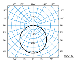
Olisq RWD4 DW 40-830 ET + Olisq RWD4 ZDR 1/2 03 TX427416
