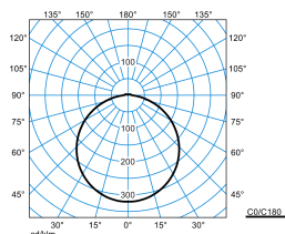
Olisq RWD4 DW 40-830 ET + Olisq RWD4 C 01 TX427011
