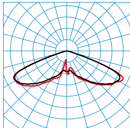
Publisca P2-RB6L-LR/2000-730 3G1S TX047856 ■ C0 - C180 ■ C90 - C270 DIN 5040: A20 UTE: 1,00 J DLOR: 100 % ULOR: 0 % CEN Flux Code: 20 57 98 100 100
