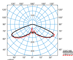
Publisca P2-RB6L-LR/2000-730 3G1S ET (CLO end value)
