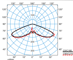
Publisca P2-RB6L-LR/2000-730 3G1S ET (CLO initial value)
