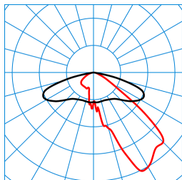
Publisca P1-AB2L-LR/3500-740 4G1S ET (CLO initial value) TX300319 ■ C0 - C180 ■ C90 - C270 DIN 5040: A30 UTE: 1,00 G DLOR: 100 % ULOR: 0 % CEN Flux Code: 35 73 97 100 100
