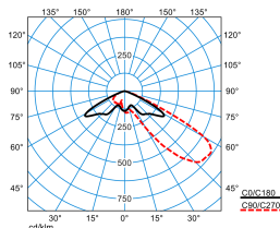
LnPlus 40-AM19L-LR/2200-740 2G1 ET (CLO initial value) TX377718
