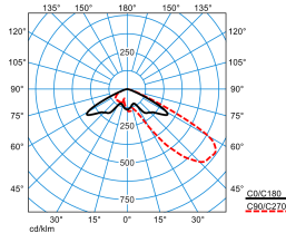
LnPlus 40-AM19L-LR/2200-740 2G1 ET (CLO end value) TX377621
