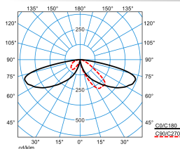
LTX KT-AB2L-LR/1200-730 2G1 ET
