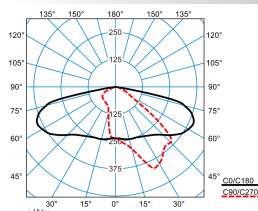
LIQ 50-AB2L-LR/3500-730 4G1S ET
