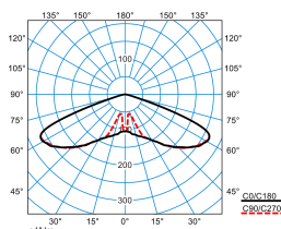
Publisca P1-RB6L-LRA/1350-730 2G1S ET (CLO end value) TX300713
