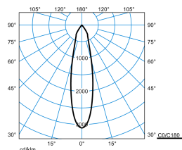
E-Line PRO 78 BV G2 RF-MF 20-830 M33 ET 05 05
