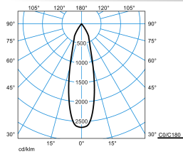
SisC 2Z RF-MF 2x50-830 M33 ETBLE 01
