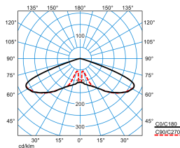
Publisca P1-RB6L-LRA/1100-740 2G1S ET (CLO initial value)
