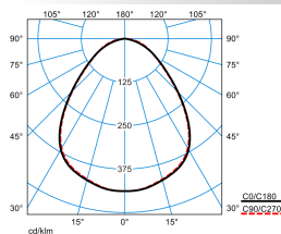
E-Line PRO 78IP50 MironaF B 200-840 ETDD L150 01 ESG 01 (LEO2)
