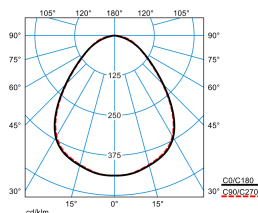
E-Line PRO 78IP50 MironaF B 200-840 ETDD L150 01 ESG 01 (LEO1)
