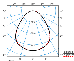
E-Line PRO 78IP50 MironaF B 200-840 ETDD L150 01 ESG 01 IP50 (LEO1)
