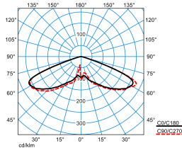
Publisca P2-RB6L-LR/2000-740 3G1S ET (CLO initial value)
