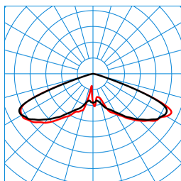
Publisca P2-RB6L-LR/2000-740 3G1S ET (CLO initial value) TX300464 ■ C0 - C180 ■ C90 - C270 DIN 5040: A20 UTE: 1,00 J DLOR: 100 % ULOR: 0 % CEN Flux Code: 20 57 98 100 100
