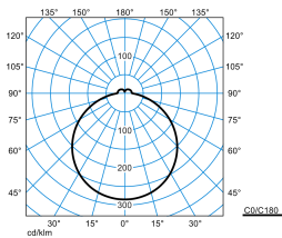
Olisq RWD2 DW 40-8TW ETDD8 PC (DSU)
