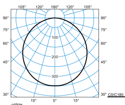
Olisq RWD2 DW 40-8TW ETDD8 PC + RWD2 ZDR 1/1 01 (DWW)
