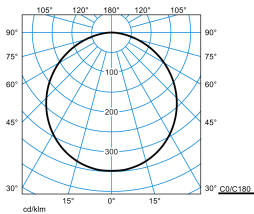
Olisq RWD2 DW 40-8TW ETDD8 PC + RWD2 ZDR 1/1 03 (DCW)
