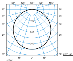
Olisq RWD2 DW 40-8TW ETDD8 PC + RWD2 ZDR 1/1 05 (DWW)
