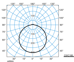
Olisq RWD2 DW 14-40/4/ML-840 ET + Olisq RWD2 ZDR 1/2 01 (stage 2)
