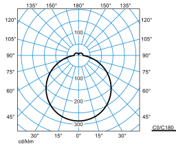
Olisq RWD2 DW 14-40/4/ML-840 ET (stage 1)
