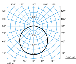
Olisq RWD2 DW 14-40/4/ML-840 ET + Olisq RWD2 C 01 (stage 2)
