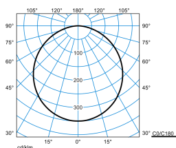
Olisq RWD2 DW 14-40/4/ML-840 ET + Olisq RWD2 ZVF 03 (stage 1)
