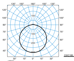
Olisq RWD2 DW 14-40/4/ML-840 ET + Olisq RWD2 ZDR 1/2 05 (stage 3)
