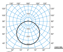
Olisq RWD2 DW 14-40/4/ML-840 ET + Olisq RWD2 C 01 (stage 3)
