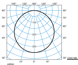
Olisq RWD2 DW 14-40/4/ML-840 ET + Olisq RWD2 ZVF 01 (stage 4)
