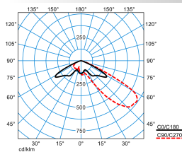
LnPlus 70-AM19L-SLR3/62000-740 48G1 ET (CLO initial value)
