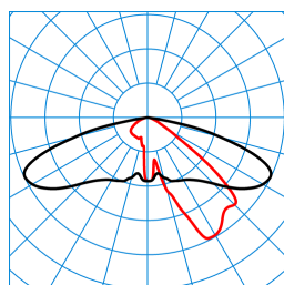
Publisca P1-AB2L-LRA/5100-740 6G1S ET (CLO initial value) TX301159 ■ C0 - C180 ■ C90 - C270 DIN 5040: A30 UTE: 1,00 G DLOR: 100 % ULOR: 0 % CEN Flux Code: 35 74 97 100 100
