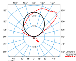
Luceos S G3 PAW-IA 170-9TW ETDS KL 01 (DS)
