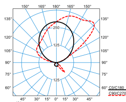
Luceos S G3 PAW-IA 170-9TW ETDS KL 01 (DCW)
