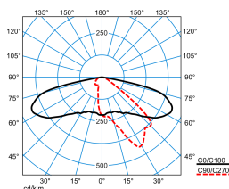
Cuvia60-AB2L12S3-135-722-ET-CAB-26 (CLO end value)
