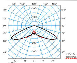
Publisca P1W-RB6L-LR/4600-730 6G1S ET (CLO initial value)
