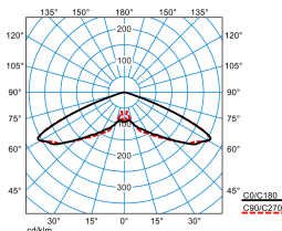
Publisca P1W-RB6L-LR/4600-730 6G1S ET (CLO end value) TX301285
