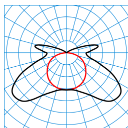
AragF 12 PXW 20-65/16ML-840 ET (stage 11) ■ C0 - C180 ■ C90 - C270 TX770568
