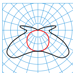
AragF 12 PXW 20-65/16ML-840 ET (stage 10) ■ C0 - C180 ■ C90 - C270 TX769760
