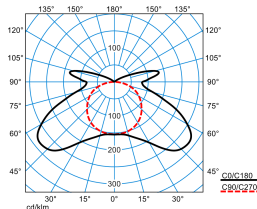
AragF 12 PXW 20-65/16ML-840 ET (stage 11) TX770568
