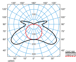
AragF 12 PXW 20-65/16ML-840 ET (stage 12) TX770023
