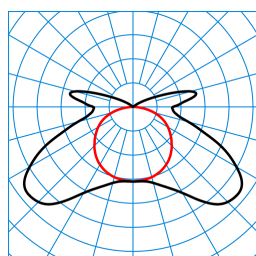
AragF 12 PXW 20-65/16ML-840 ET (stage 12) ■ C0 - C180 ■ C90 - C270 TX770023
