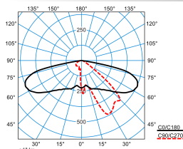
Publisca P2-AB2L-LRA/2200-740 3G1S
