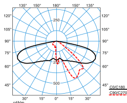
Publisca P2-AB2L-LRA/2200-740 3G1S ET (CLO initial value)
