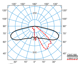
Publisca P2-AB2L-LRA/2200-740 3G1S ET (CLO end value)
