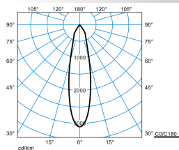
E-Line PRO 78 BV G2 RF-MF 50-835 M34 ET 05 Blank
