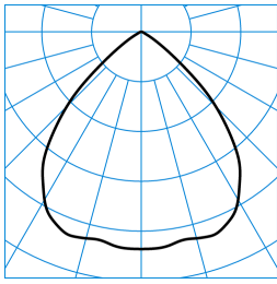
InperlaL G2 C07 BR22 2700-840 03 + RG-PC ■ C0 - C180 TX052927
