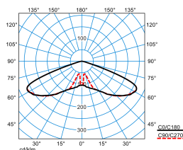
Publisca P2-RB6L-LR/1800-740 2G1S
