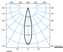
7651 LentyP L-SP 30-835 M34 ET 03 (225)
