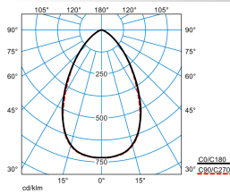
Mirona Fit 4L TB 260-840 ETDD+LLWS IS3 TX771309
