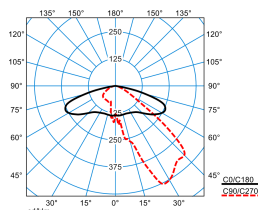
Publisca P2-AB2L-LR/2900-730 4G1S ET (CLO end value)
