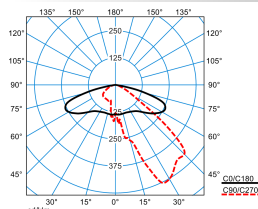
Publisca P2-AB2L-LR/2900-730 4G1S ET (CLO initial value)
