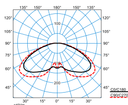
Publisca P1W-RBT-LR/3800-740 6G1S ET (CLO initial value)
