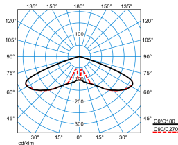
Publisca P2-RB6L-LRA/1350-740 2G1S
