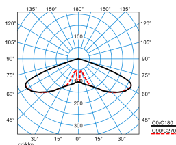
Publisca P2-RB6L-LRA/1350-740 2G1S ET (CLO end value)
