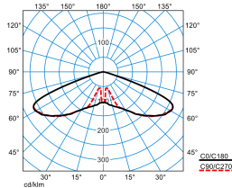
Publisca P2-RB6L-LRA/1350-740 2G1S ET (CLO initial value)
