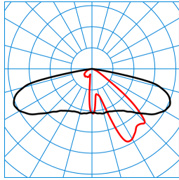
Publisca P2-AB2L/1200-740 2G1S TX047699 ■ C0 - C180 ■ C90 - C270 DIN 5040: A30 UTE: 1,00 G DLOR: 100 % ULOR: 0 % CEN Flux Code: 34 70 96 100 100
