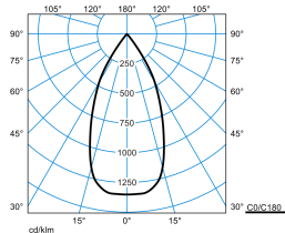
E-Line PRO 78 BV G2 RF-WFL 50-827 M32 ET 03 Blank
