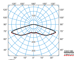
7650 L-SLB 24V Inotec L37 05 (150)
