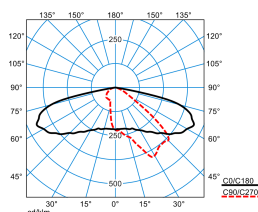
LIQ 50N-AB2L-LR/1650-740 2G1 ET (CLO end value)
