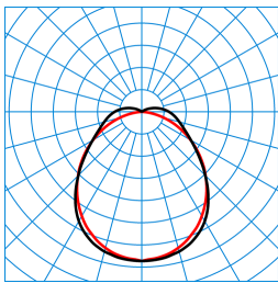
OleveonF 15 L 6000-840 ETDD PC +HFS TX770819
