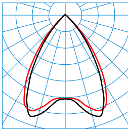
Ondo G2 LW 22000-840 ETDD + Reflector PC 12-22 TX782726
