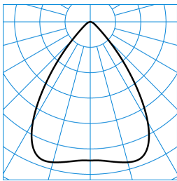
Ondo G2 LW 22000-840 ETDD TX784077
