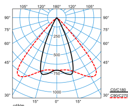
E-Line PRO 78 Grado WRS-DF84 20-EC M47 ET 05 Blank
