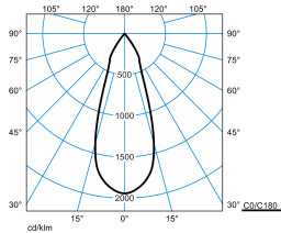
E-Line PRO 78 BV G2 RF-FL 50-827 M32 ETDD 03 Blank
