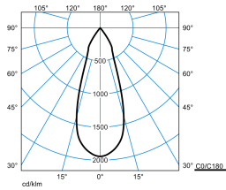
E-Line PRO 78 BV G2 RF-FL 50-827 M32 ETDD 03 03
