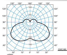
PolaronIQ WD1-2 LED3000-840 ET TX773891
