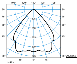
InperiaLP C05 HR22 1000-840 03 + DA 01 TX041689
