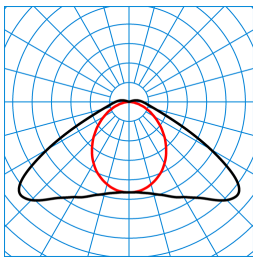
Nextrema G3 XB 23-840 ETDD TWP PC TX768590
