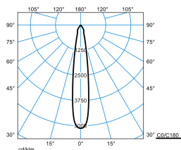
E-Line PRO 78 BV G2 RF-SP 30-EC M39 ET 05 Blank
