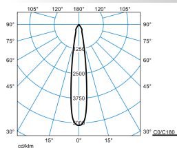
E-Line PRO 78 BV G2 RF-SP 30-EC M39 ET 05 05
