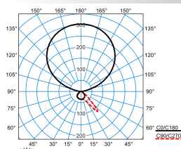
Luceos S BS G3 PAW-IL 125-8TW ETDS FU 01 (DWW)
