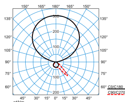
Luceos S BS G3 PAW-IL 125-8TW ETDS FU 01 (DSU)
