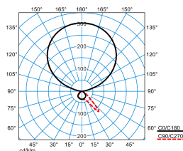
Luceos S BS G3 PAW-IL 125-8TW ETDS FU 01 (DCW)
