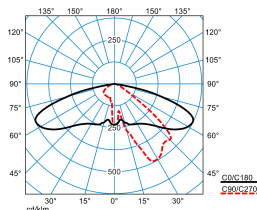
Publisca P1-AB2L-LR/4600-730 6G1S ET (CLO end value)
