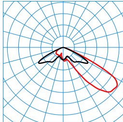
LnPlus 40-AM19L-SLR1/10000-730 8G1 ET (CLO end value) TX377076
