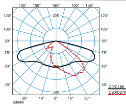
Jovie 70-AB7L-8-100-730-CLO-B
