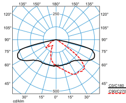
Jovie 70-AB7L-8-100-730-CLO-E
