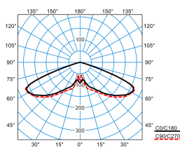
Publisca P2-RB6L-LRA/3500-740 4G1S ET (CLO end value)
