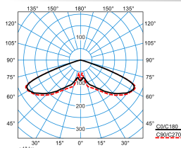
Publisca P2-RB6L-LRA/3500-740 4G1S ET (CLO initial value)
