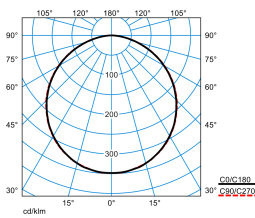
Olisq QWD2 DW 20-840 ET IK + Olisq QWD2 ZDR 1/1 03 TX460801
