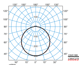
Olisq QWD2 DW 20-840 ET IK + Olisq QWD2 ZDR 1/2 01
