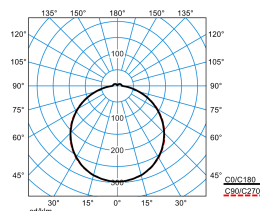
Olisq QWD2 DW 20-840 ET IK + Olisq QWD2 ZDR 1/2 05
