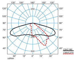
Jovie 50-AB2L-6-68-740-CLO-B
